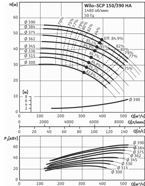
Wilо-SCP 150/390 HA
