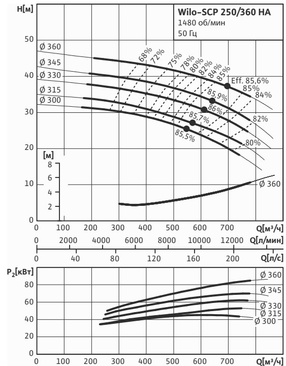
Wilо-SCP 250/360 HA
