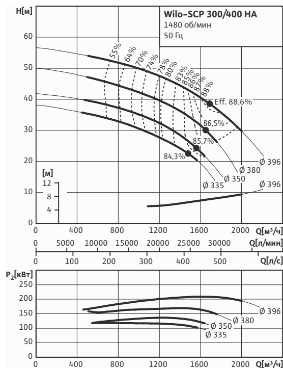
Wilо-SCP 300/400 HA
