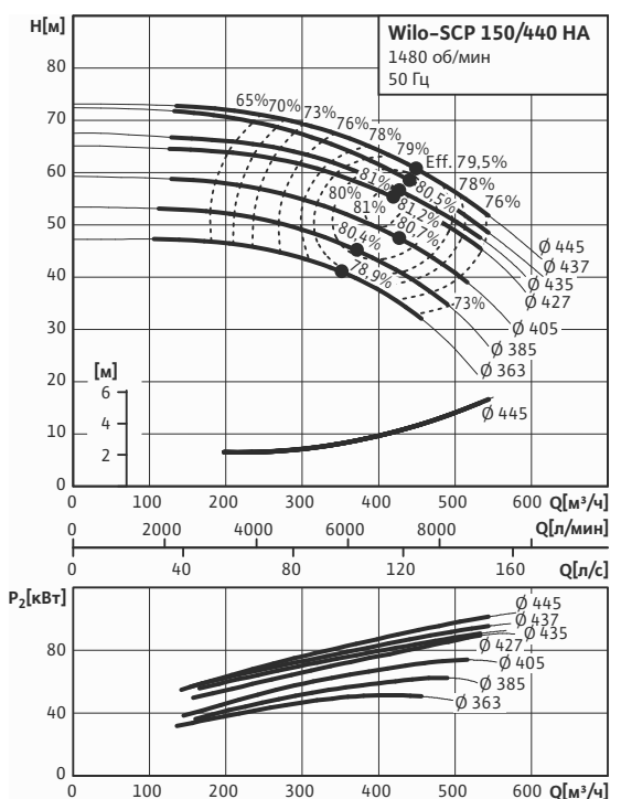
Wilо-SCP 150/440 HA
