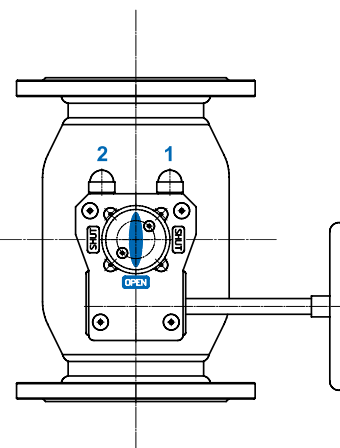
Редуктор в положении «ОТКРЫТО»
