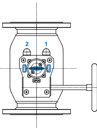
Редуктор в положении «ЗАКРЫТО»
