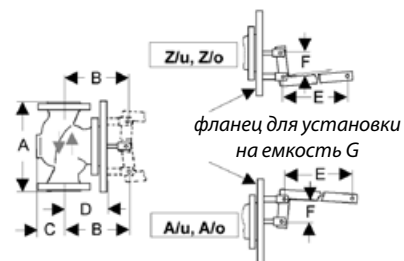
NV55e
