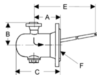
NV71 Z/u
