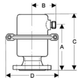
EB1.12 DN 65–100
