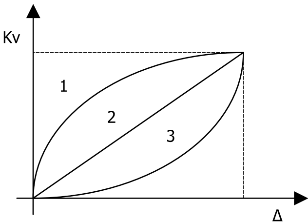
1 – характеристика запорного плунжера 2 – линейная характеристика 3 – квадратичная характеристика
