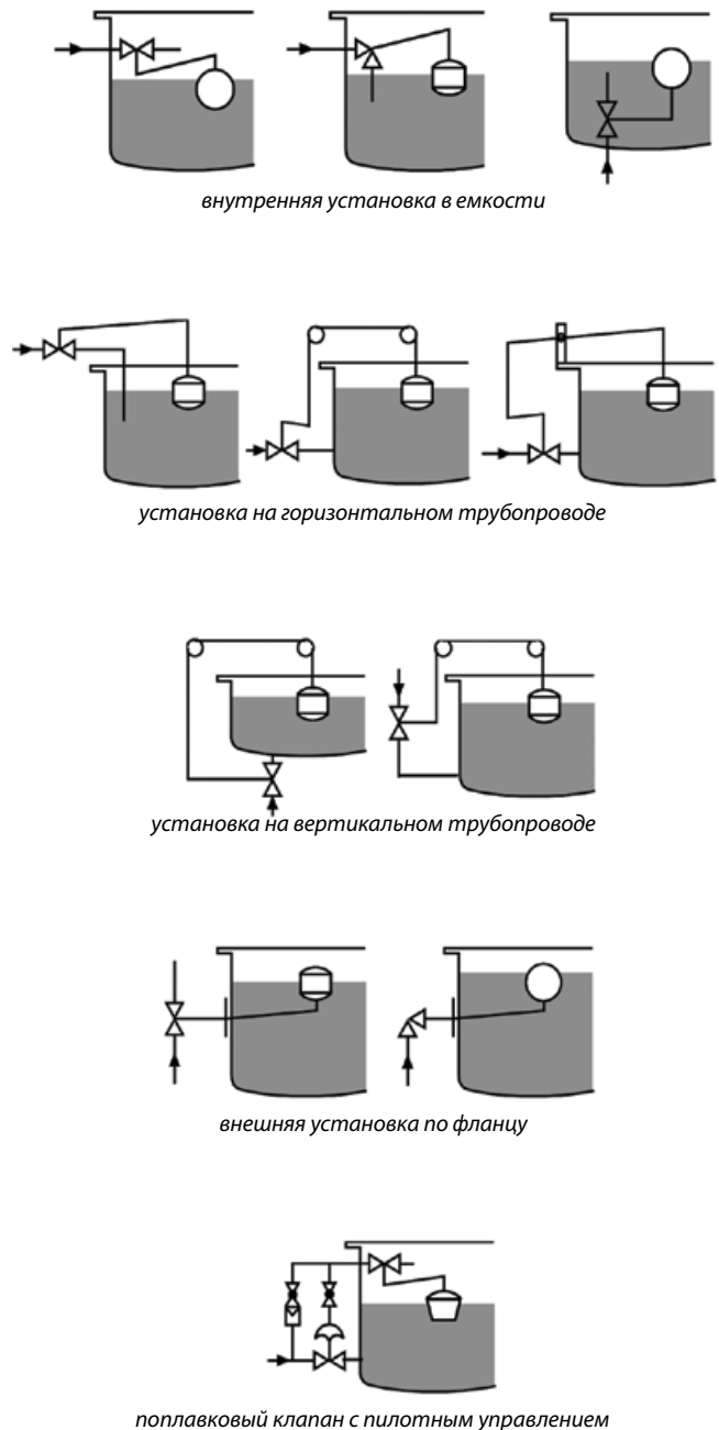
Рис. 1. Примеры установки поплавковых клапанов
