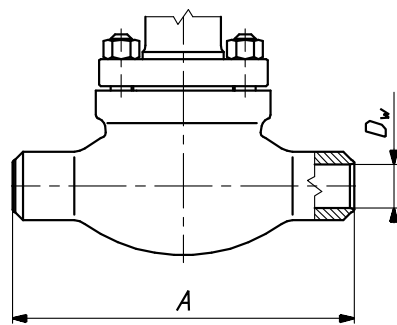
сварное присоединение
