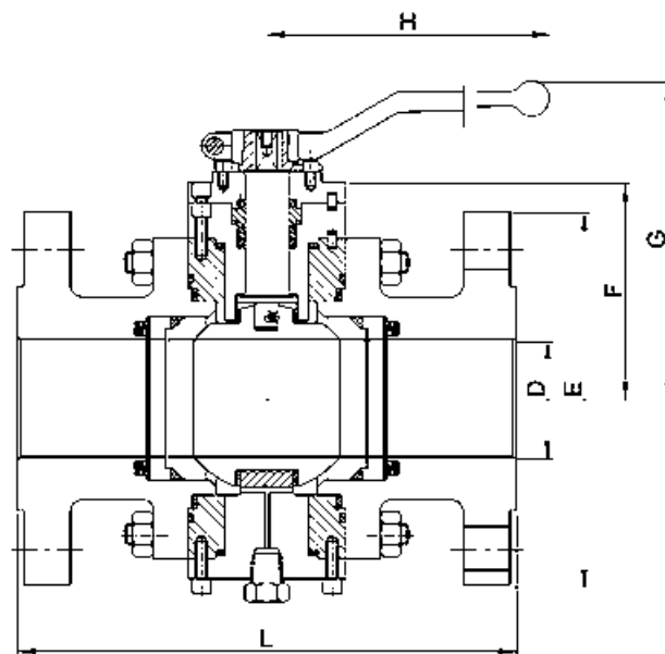
Конструкция крана с двумя опорами шара
