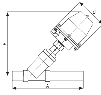
PP1040/PP1041
