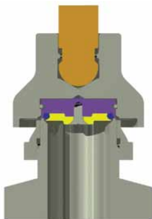
Мягкое уплотнение
