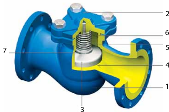
Серия 287
