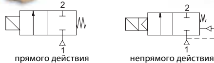
Нормально закрытые
