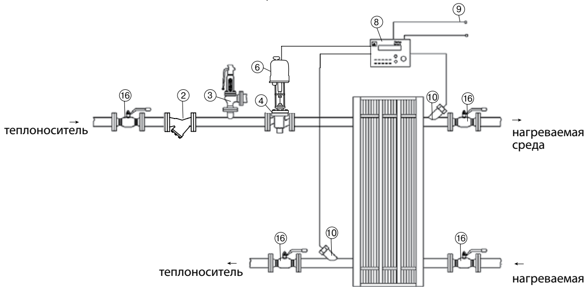
Водо-водяные ТО
