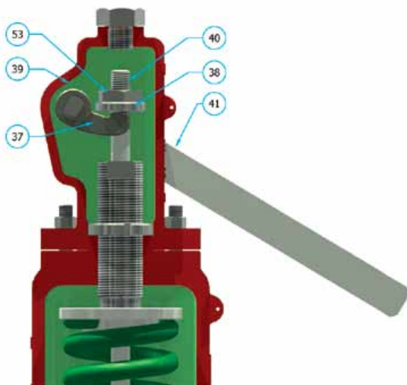
Подрывной рычаг
