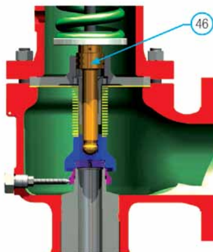
Сифонно-плунжерный клапан
