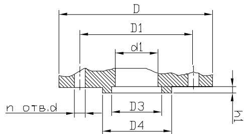
Исполнение 8
