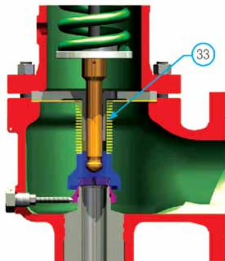
Сифонный клапан
