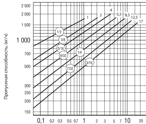
Перепад давлений, МПа × 10 -1 , (бар) Модель 883
