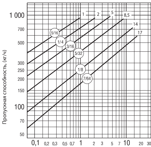
Перепад давлений, МПа × 10 -1 , (бар) Модель 882
