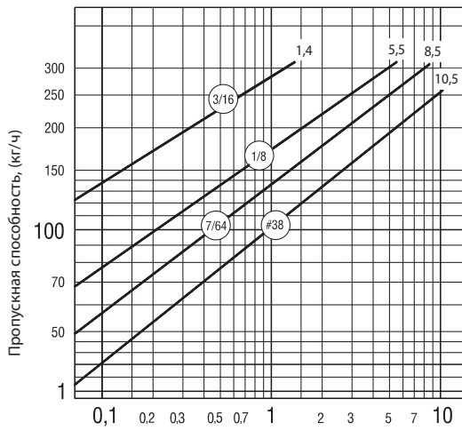
Перепад давлений, МПа × 10 -1 , (бар) Модель 880
