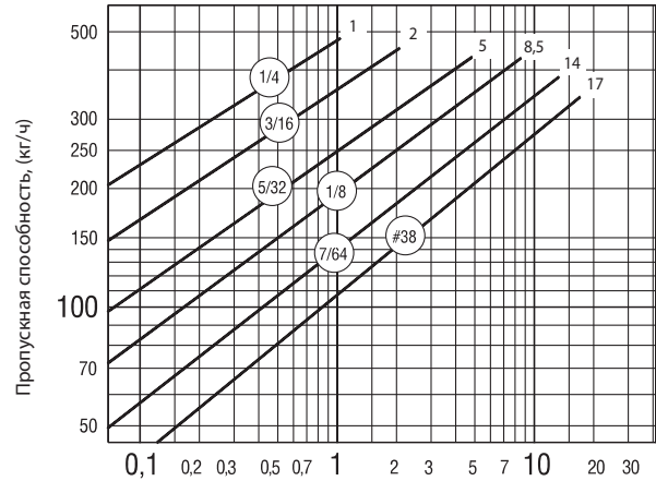
Перепад давлений, МПа × 10 -1 , (бар) Модель 881
